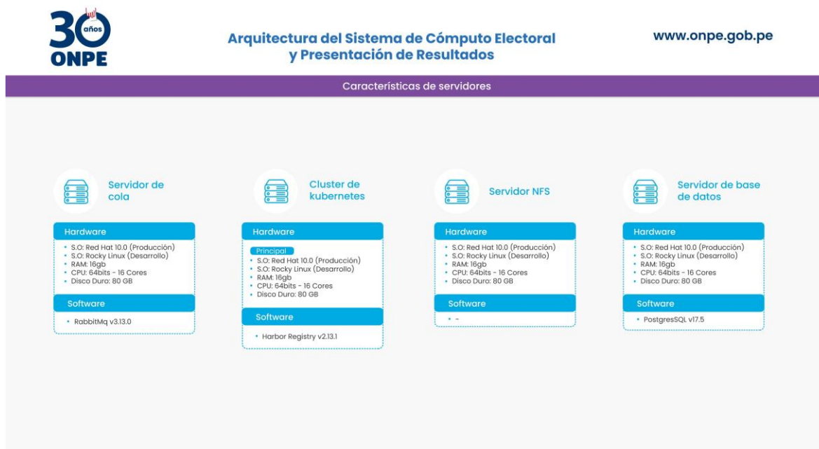
Ilustración 6. Características de Hardware y Software del Sistema de Cómputo Electoral
