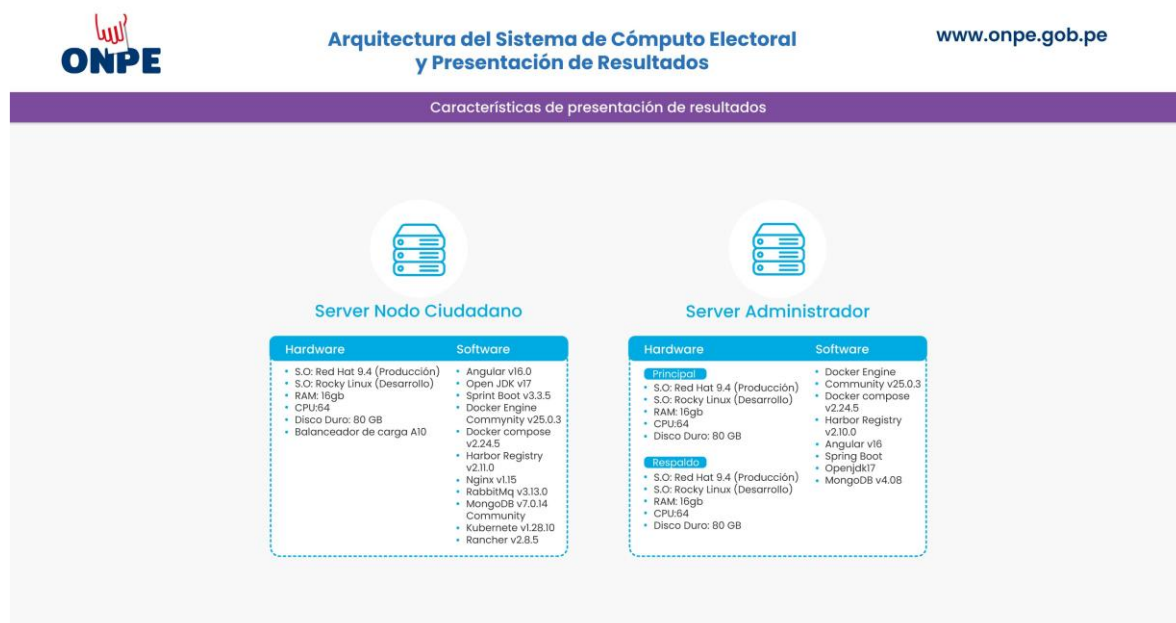
Ilustración 12. Características de Hardware y Software del Sistema de Cómputo Electoral
