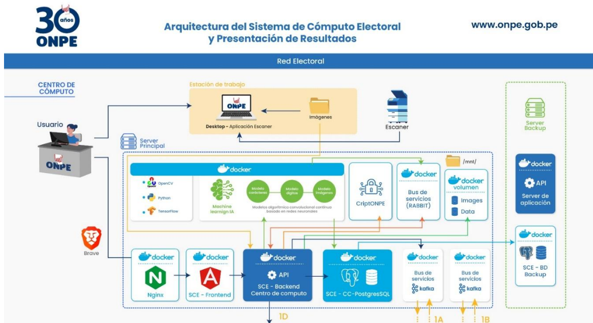
Ilustración 8. Arquitectura de los componentes en el Centro de Cómputo del Sistema de Cómputo Electoral.
