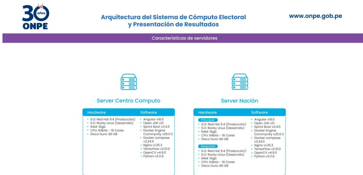
Ilustración 5. Características de Hardware y Software del Sistema de Cómputo Electoral
